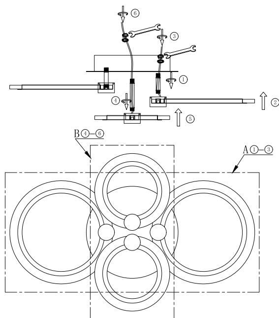
Монтажный чертеж потолочного светильника ELEGANT BLISS 120Вт
