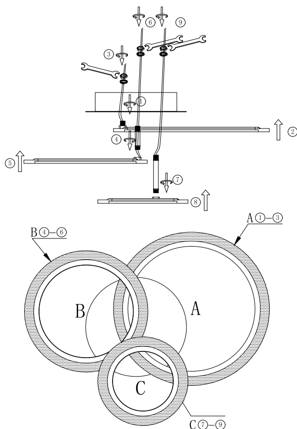
Монтажный чертеж потолочного светильника ELEGANT BLISS 60Вт
