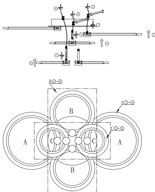
Монтажный чертеж потолочного светильника ELEGANT BLISS 120Вт
